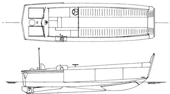
Mk1 (madera)
