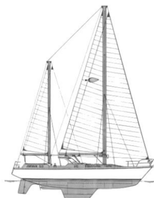
A77 Almansa tipo Mango 52'
